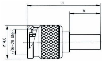
TNC Kabelstecker - Crimp (schematisch)
