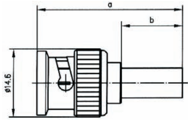
BNC Kabelstecker - Crimp (schematisch)
