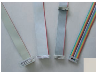
HDD Festplattenkabel Ultra ATA 133 Kabel SCSI Flachbandkabel u. a.
