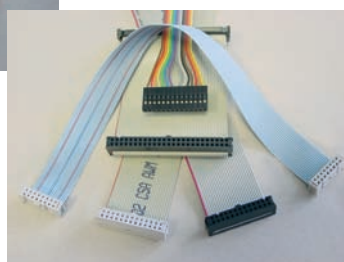
HDD Festplattenkabel Ultra ATA 133 Kabel SCSI Flachbandkabel u. a.
